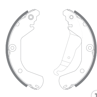
2733-CPA Ø230 x 41mm
